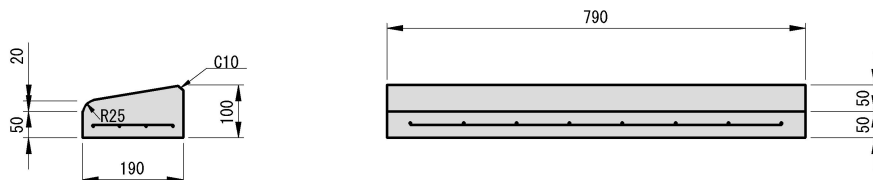
特殊B変形 190 × 100 × 790 30 kg
