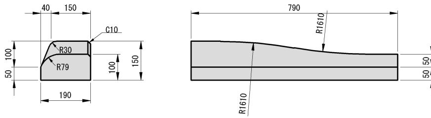
B変形 190 × 100 × 790 34 kg
