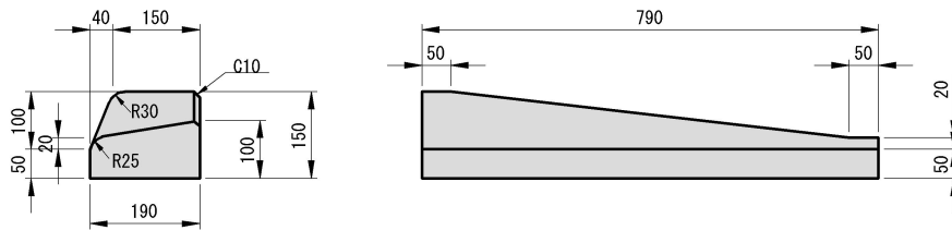
特殊B変形 190 × 100 × 790 30 kg
