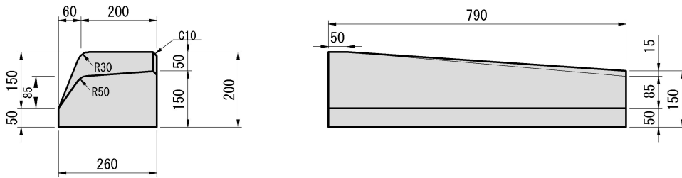
特殊A変形1 200/260×150/200×790 75 kg
