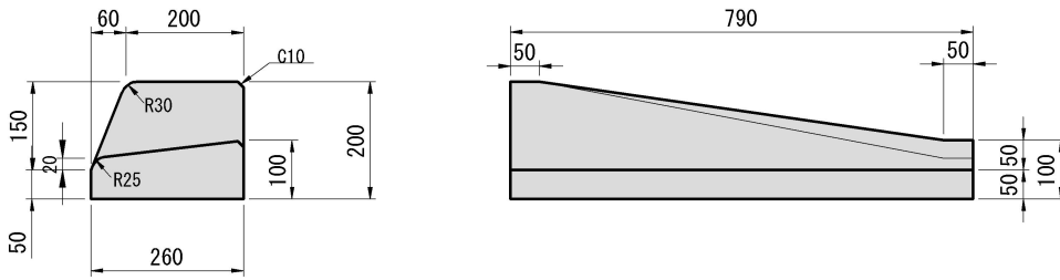
特殊A変形1段 200/260×100/200×790 64 kg
