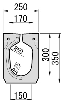
正面図
