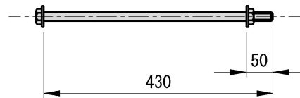
組立用ボルト M16×430 亜鉛メッキ製
