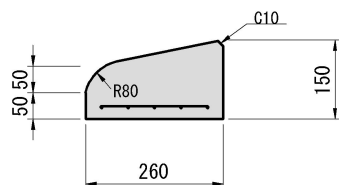
B 変形 260 × 150 × 790
