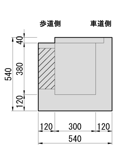
側面図
