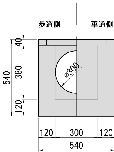
側面図
