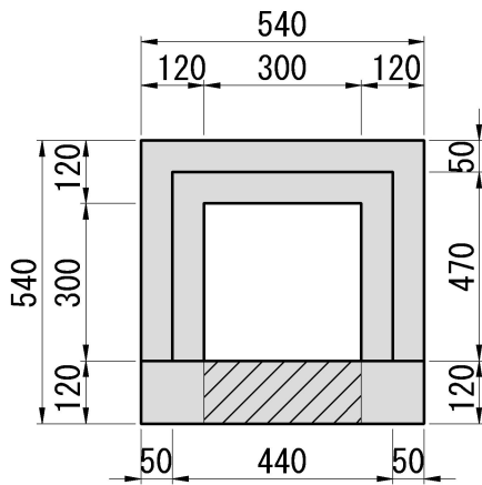
側面図
