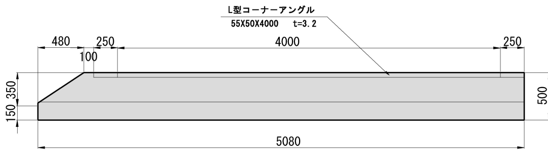
平面図
