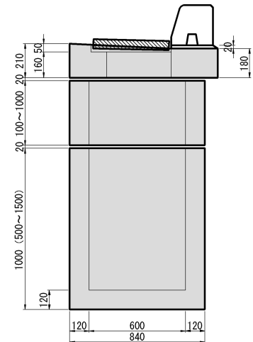
組合図2
