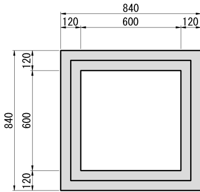
下部及び中間部平面図
