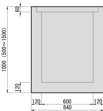
下部側面図
