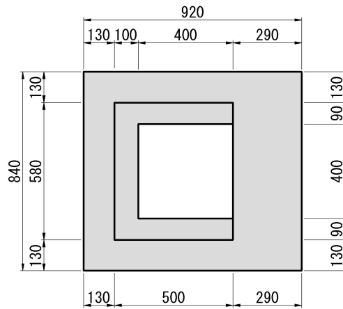
上部側面図
