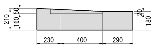
上部側面図
