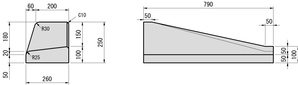
特殊 A 変形1段 200/260 × 100/250 × 790 72 kg
