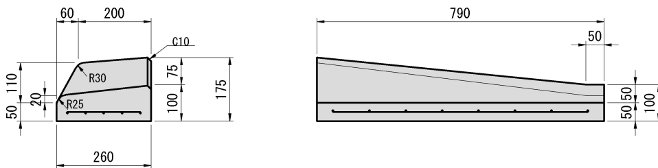
特殊 A 変形2 200/260 × 100/175 × 790 55 kg
