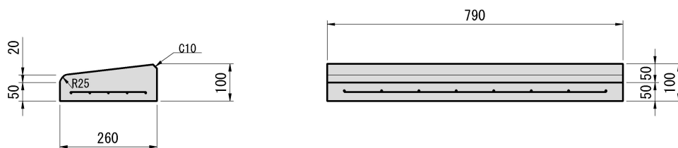
特殊 B 変形 260 × 100 × 790 41 kg
