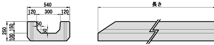
横断溝 B型
