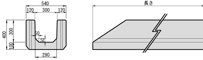
横断溝 A型
