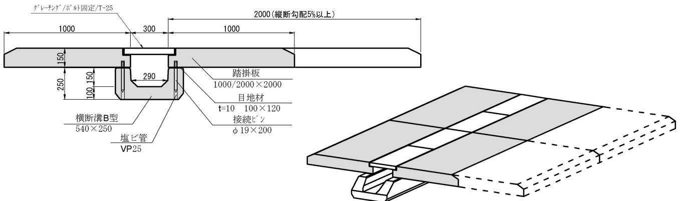
組合せ図 (B型)
